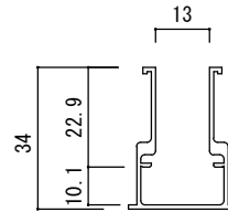
M12ロック機能付アルミレール
